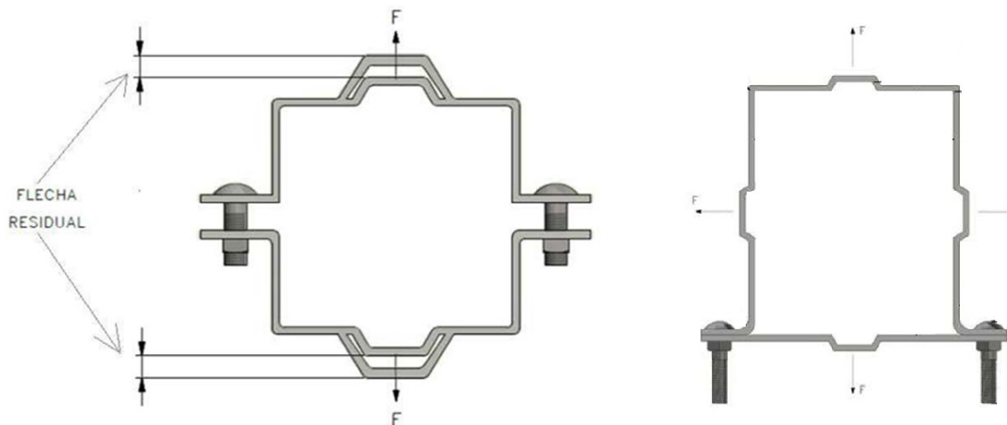
Figura 3 - Detalhes para Ensaio
