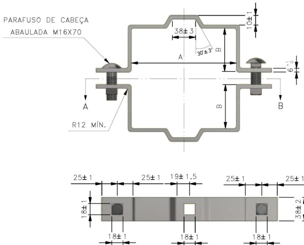
Figura 1 - Cinta para poste duplo T - tipo 1
